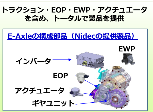
EOP：電動オイルポンプ、EWP：電動ウォーターポンプ 27
