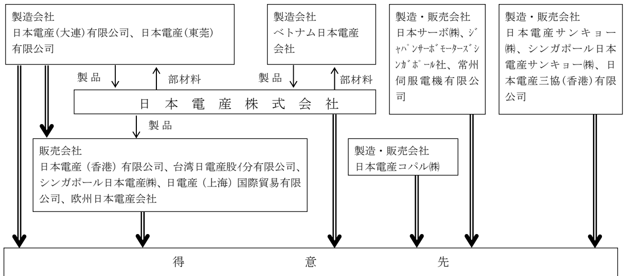
(中型モータ)
