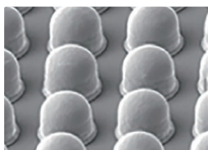
■ Cu pillar
