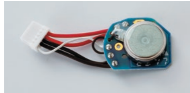
■振動モーター + 基板 型式: LAV10C-001 用途: アラーム 特長: 高寿命・高信頼性
