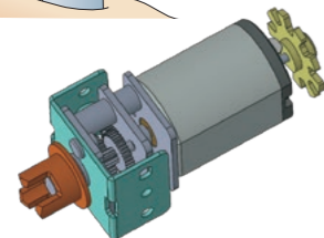
■ギヤブロック 型式: LA12GE-344SF (モーター+ギヤブロック) 用途: モーターの回転で薬剤を押し出して注入する
