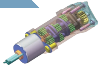
■ステッピングモーター + ギヤ 型式: LPD6G 用途: 自動注射器(薬剤投与) 特長: 高寿命・高信頼性制御性
